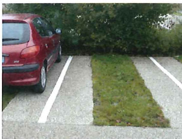
bande de roulement béton et gazon
